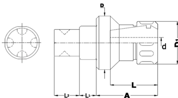
Modular Extension ER Collet Chuck (mm)
